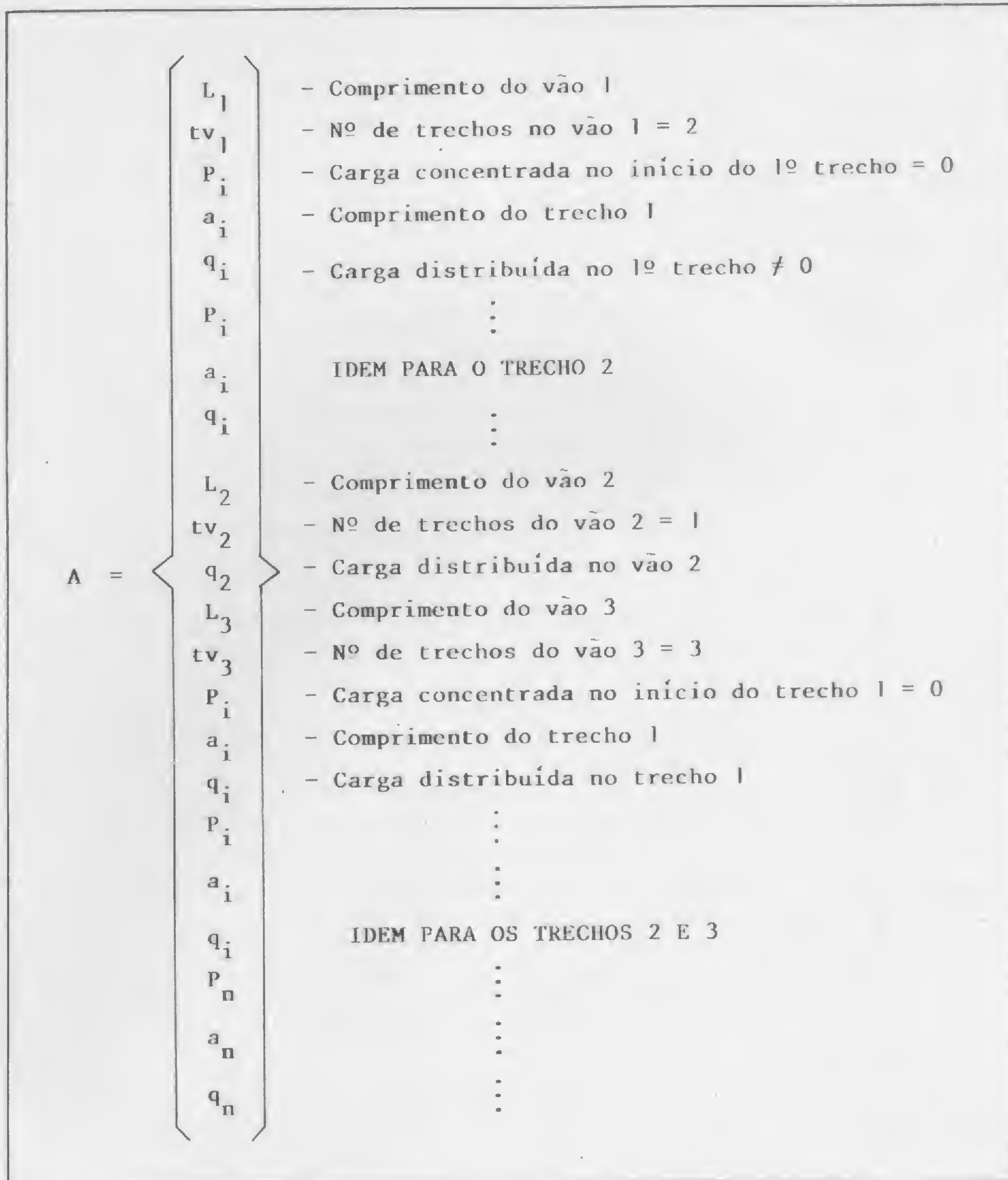
Figura 2 – Estrutura do vetor de trabalho
